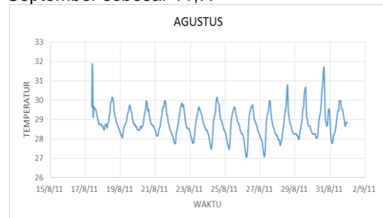
Gambar 4.4 Karakteristik SPL Agustus 2011 Stasiun 01
