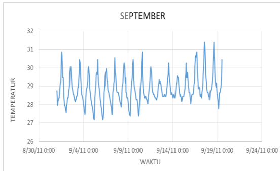
Gambar 4.5 Karakteristik SPL bulan September 2011 stasiun 01
