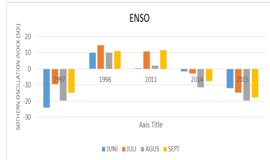
Gambar 4.3 Southern Oscillation Index (SOI) periode Juni – September pada tahun 1997 – 1998, 2011, 2014 – 2015
