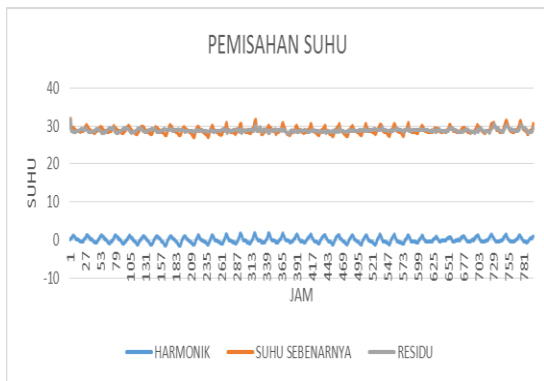
Gambar 4.13 Suhu harmonik, suhu sebenarnya dan suhu residu (non harmonik) Stasiun 02
