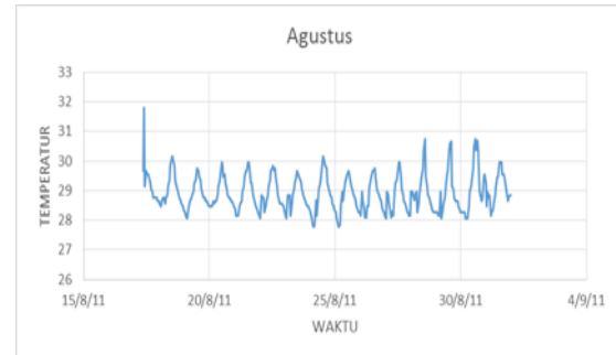
Gambar 4.11 Karakteristik SPL Agustus 2011 Stasiun 02
